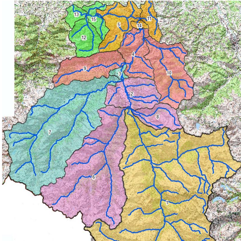
Figure 13 : Sous-bassins versants relatifs aux débits de crue de référence (SUEZ – PLVG, 2019)
