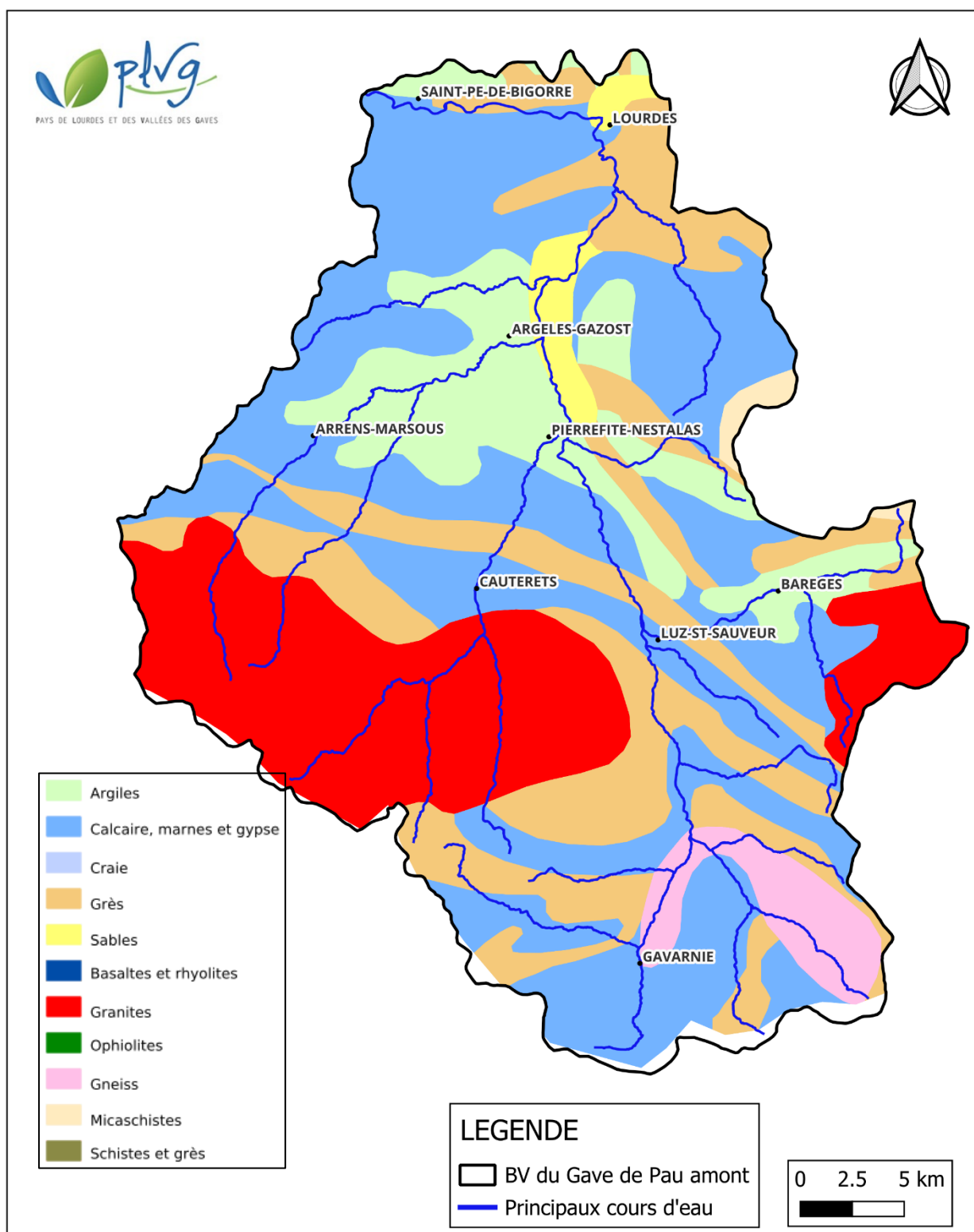
Figure 8 : Carte lithologique, PLVG 2026
