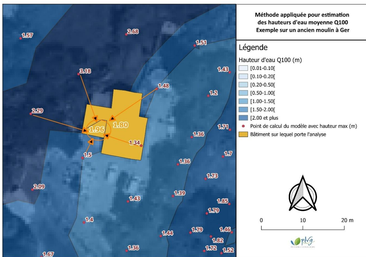
Figure 38 : Description de la méthode de calcul de la hauteur d'eau moyenne à proximité d'un bâtiment à partir des hauteurs maximales
