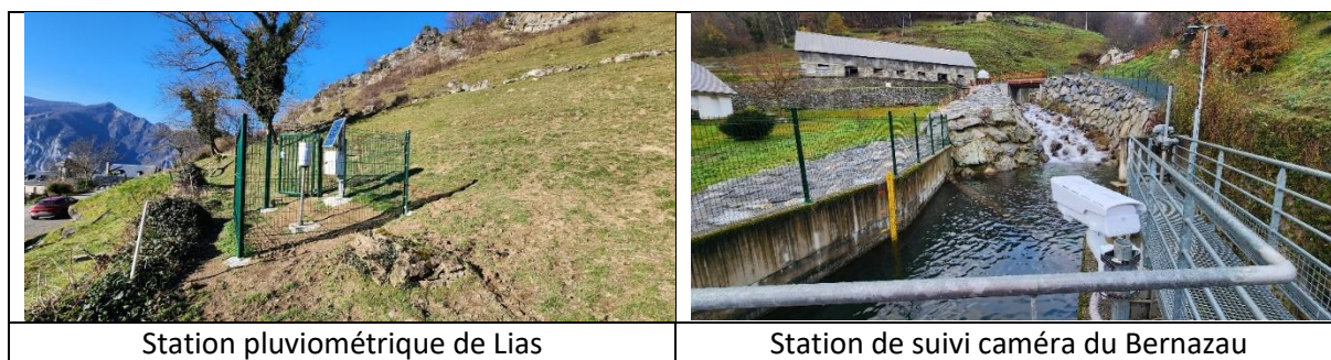
Figure 57 : Illustrations d'une station pluviométrique et d'une station avec suivi caméra
