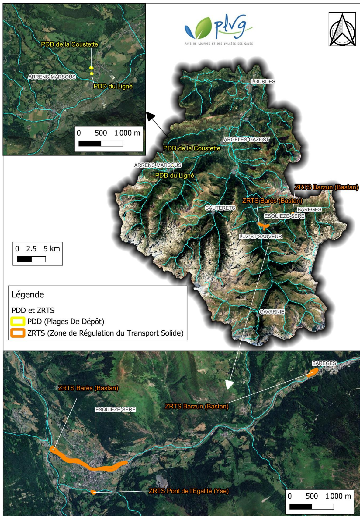
Figure 72 : Les Plages De Dépôt (PDD) et les Zones de Régulation du Transport Solide (ZRTS)
