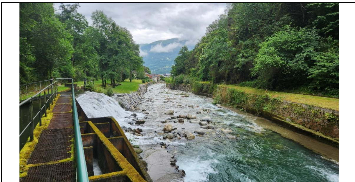
Figure 69 : Système d'endiguement du gave de Cauterets après travaux 2024 depuis le seuil du Berty
